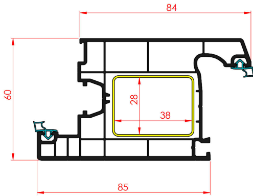
60 mm 3 odacıklı İçe Açılır Kapı Profili 60 mm 3 Chamber Inward Opening Door Profile
