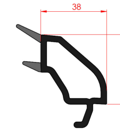
60 mm lik 4 mm Çift Cam Çıtası 60 mm 4 mm Double Glazing Bead
