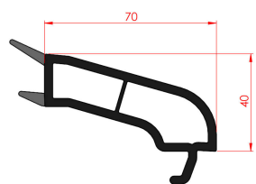
60 mm lik 4 mm Tek Cam Çıtası 60 mm 4 mm Single Glazing Bead
