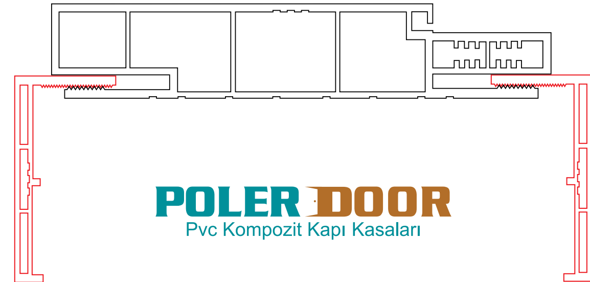
44x90 Ferli Pervaz 44x90 Ferrule Molding إطار ذو الطوق 90*44
