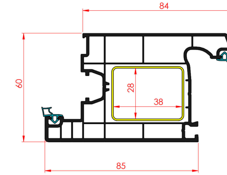
60 mm 4 odacıklı İçe Açılır Kapı Profili 60 mm 4 Chamber Inward Opening Door Profile
