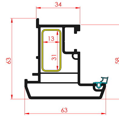
60 mm 3 odacıklı Hareketli Orta Kayıt Profili 60 mm 3 Chamber Movable Middle Registration Profile
