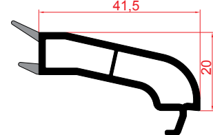
70mm Tek Cam Çıtası 70mm Single Glazing Bead لوح الزجاج مفرد 70 مم
