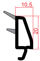
Sürme Çift Cam Çıtası Sliding Double Glazing Bead لوح الزجاج مجوز بالانزلاق
