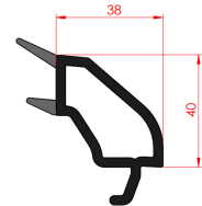
60 mm lik 4 mm Çift Cam Çıtası 60 mm 4 mm Double Glazing Bead
