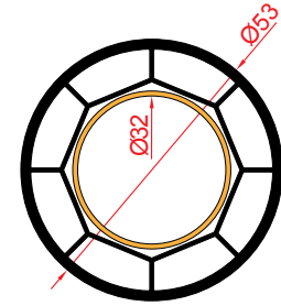
70mm Açılı Dönüş Boru Profili 70mm Angled Return Pipe Profile بروفيل أنبوب الدوران ذو الزاوية 70 مم
