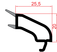
20 mm Çift Cam Çıtası 20 mm Double Glazing Bead
