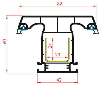
60 mm 3 odacıklı Orta Kayıt Profili 60 mm 3 Chamber Middle Registration Profile
