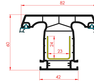
60 mm 4 odacıklı Orta Kayıt Profili 60 mm 4 Chamber Middle Registration Profile
